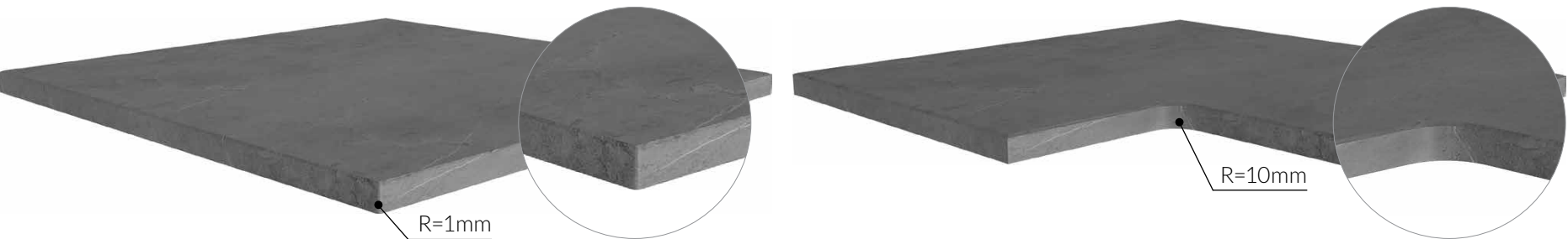
Минимальный радиус наружного закругления R=1мм The minimum radius of outer rounding R=1mm Der Mindestradius der äußeren Rundung R=1mm
