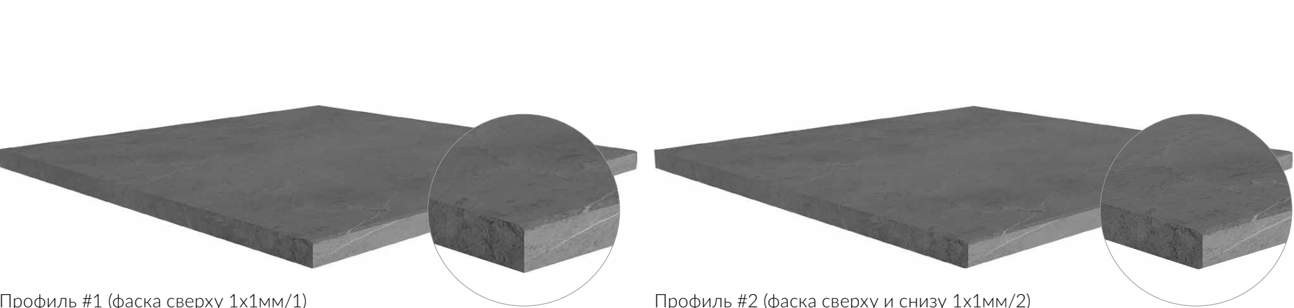
Профиль #1 (фаска сверху 1x1мм/1) Edge profile #1 (chamfer 1x1mm/1) Kantenprofil #1 (Abschrägung 1x1mm/1)
