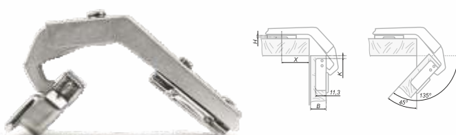
Петля 45° накладная, угол открывания 95° для ШНУ, ШЛУ, ШЛскос
