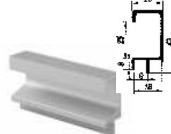
Профиль-ручка
