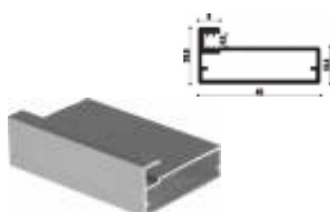
Профиль для алюминиевых фасадов Z-13
