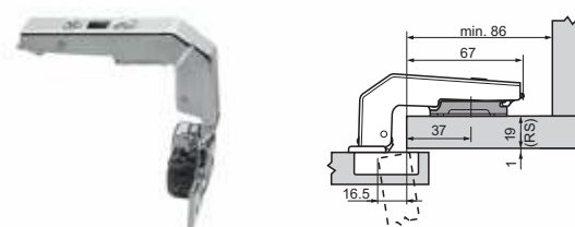
Петля ФАЛЬШПАНЕЛЬ накладная для ШЛК, ШНК (на фальш панель)
